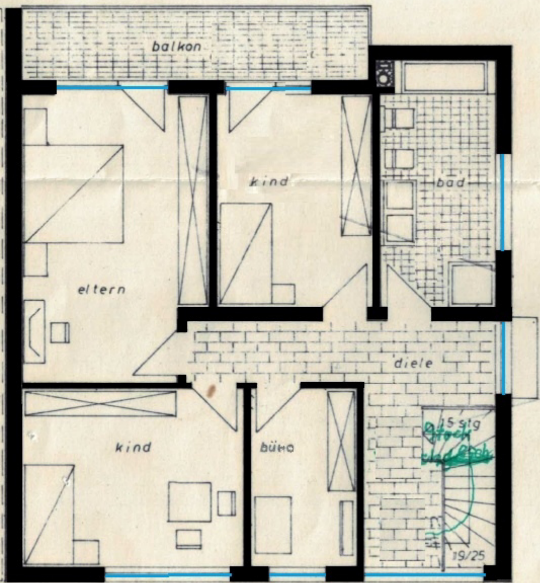
Obergeschoss
